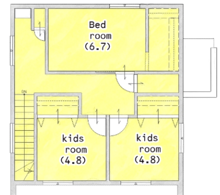
2階平面図
