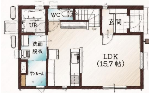
1階平面図
