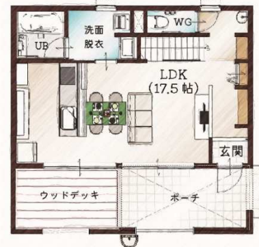
1階平面図
