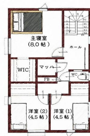
2階平面図
