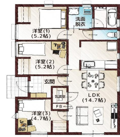
1階平面図
