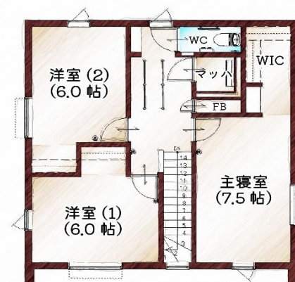
2階平面図
